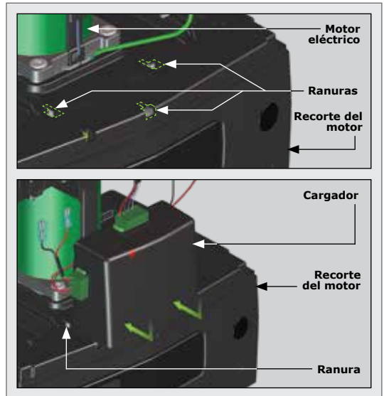
FIGURA 53. INSTALACIÓN DEL CARGADOR
