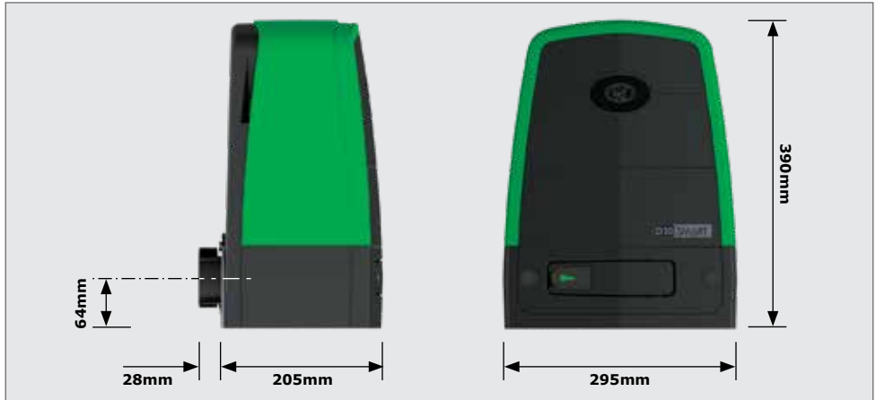
FIGURA 1. D10 SMART - D10 TURBO SMART - D20 SMART DIMENSIONES FÍSICAS
