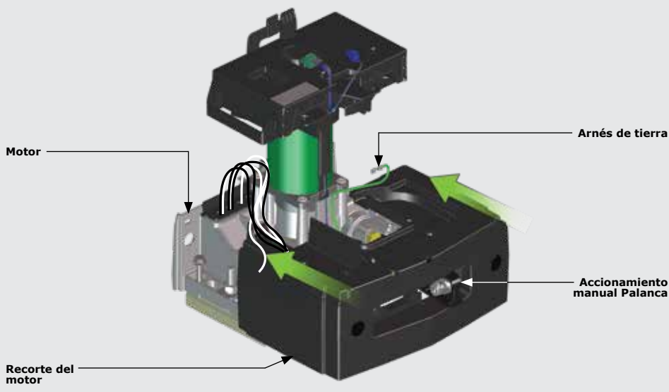
FIGURA 52. POSICIONAMIENTO DEL AJUSTE
